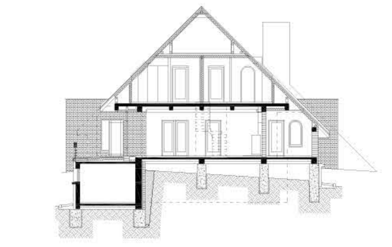
SECTIUNE CARACTERISTICA
