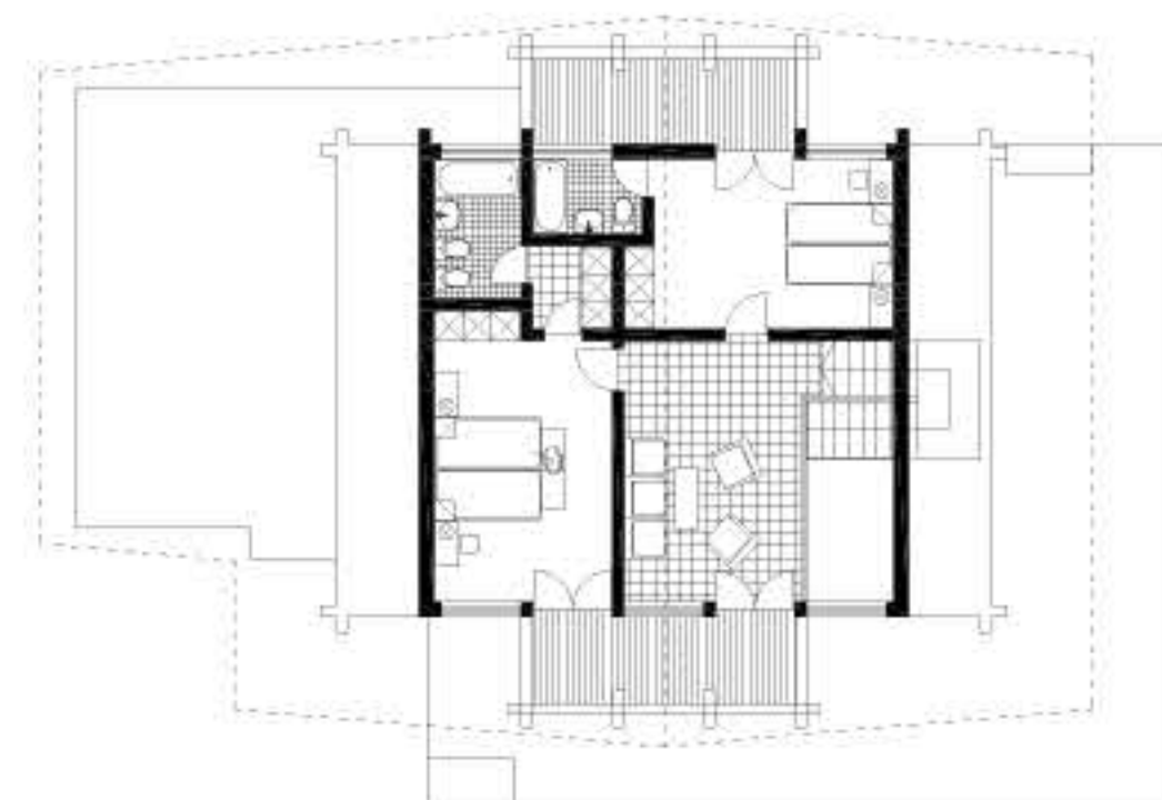
PLAN ETAJ
